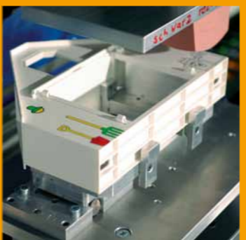
Linear-Automaton variabler Tamponaufsatzpunkt
